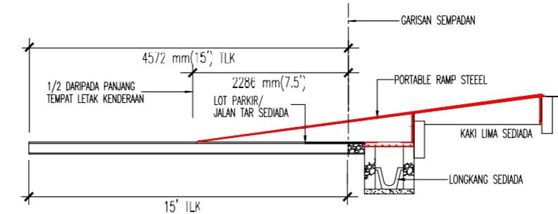
KERATAN LONGKANG 'RAMP STEEL'
