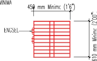
PERINCIAN KEKISI BESI
