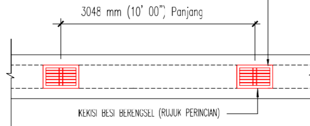
PELAN LONGKANG
