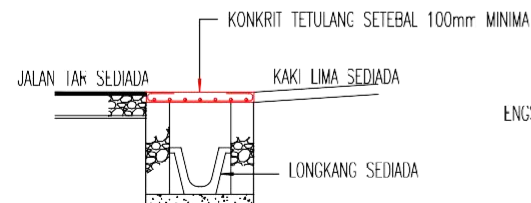
KERATAN LONGKANG
