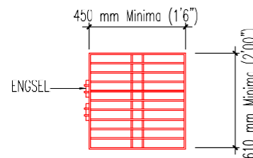
PERINCIAN KEKISI BESI
