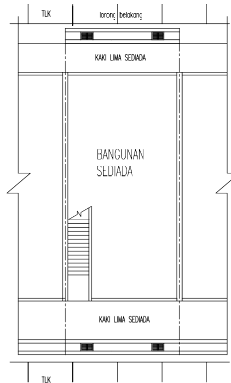
PELAN LANTAI
