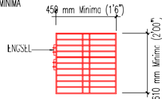
PERINCIAN KAKIS BESI
