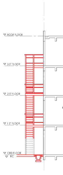
KERATAN Skala : NTC
