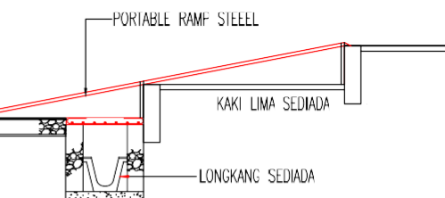
KERATAN LONGKANG 'RAMP STEEL'
