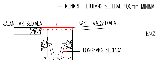
KERATAN LONGKANG
