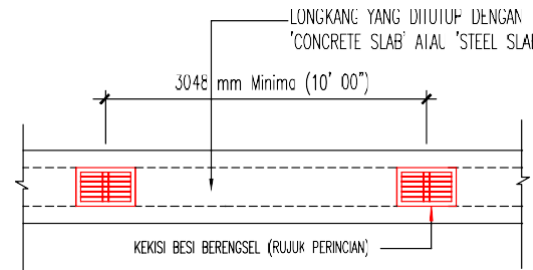
PELAN LONGKANG
