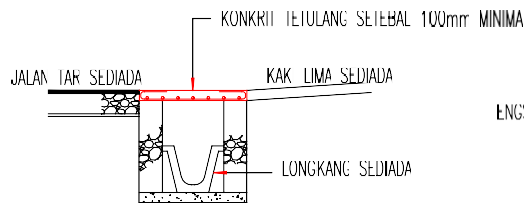
KERAJIAN LONGKANG
