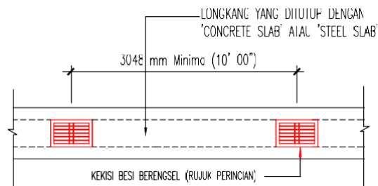
PELAN LONGKANG
