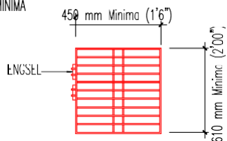
PERINCIAN KEKISI BESI
