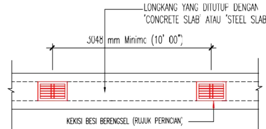
PELAN LONGKANG
