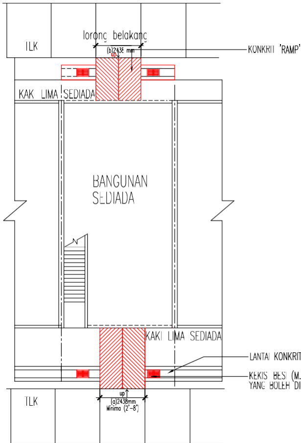
PELAN LANTAI
