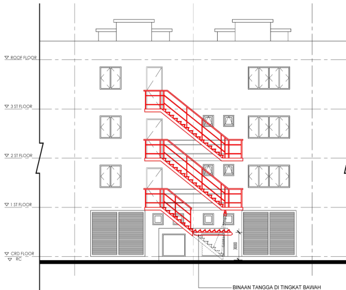
PANDANGAN SISI Skala : NTC
