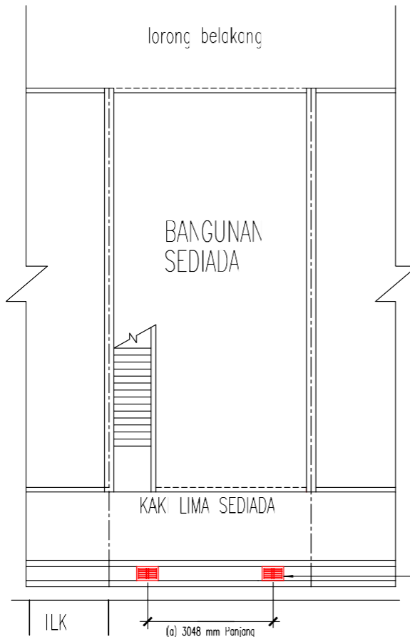
PELAN LAINA
