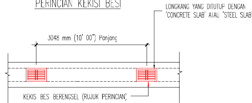
PELAN LONGKANG
