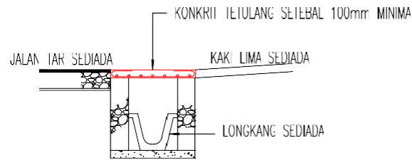
KERAJIAN LONGKANG
