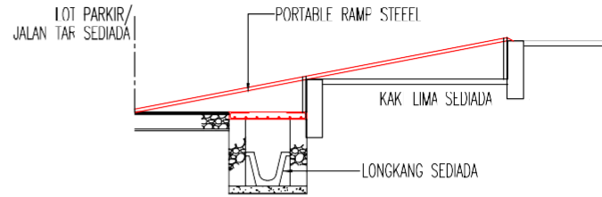
KERAJIAN LONGKANG 'RAMP STEEL'
